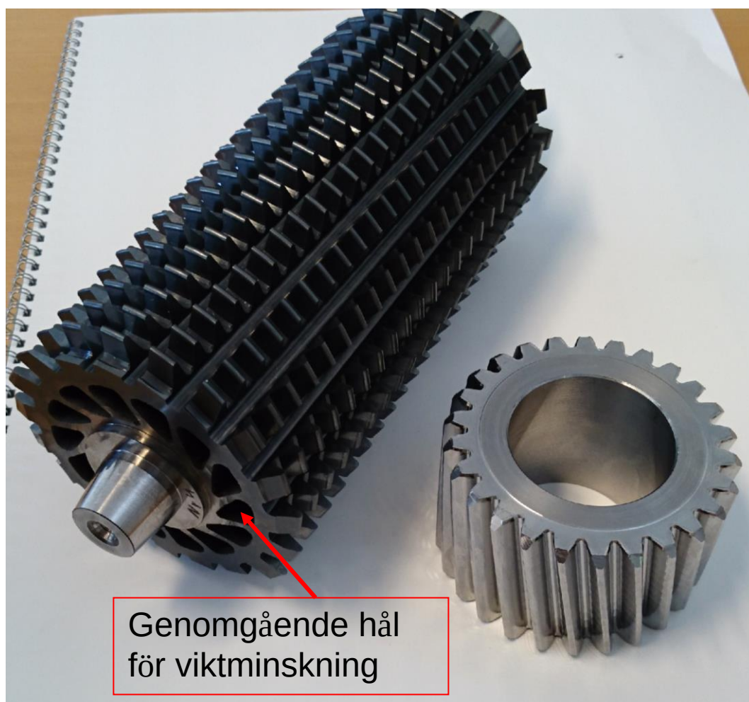
Figur 6. Additivt tillverkad snäckfräs i Vibenite®60 (med genomgående hål för viktninskning) samt det första kugghjul som tillverkats med detta verktyg. Verktuget gick full livslängd (800 kugghjul) med endast minimal förslitning och kommer att rekonditioneras och användas igen. (Verktuget är belagt).
