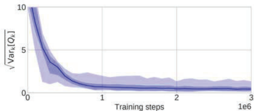
Figur 19. Den epistemiska osäkerheten minskar med antalet träningssteg (Hoel, 2021).
