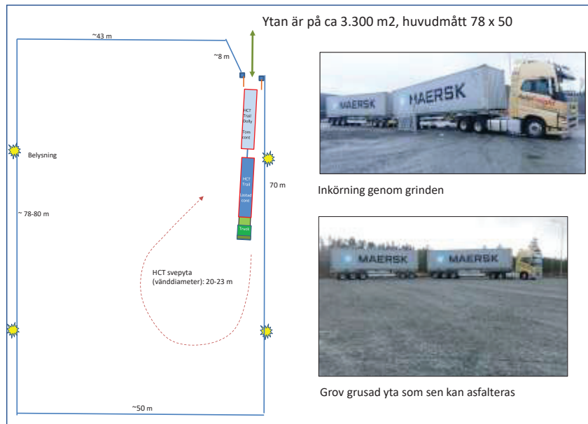
Figur 77. Dryport – Nuvarande utformning
