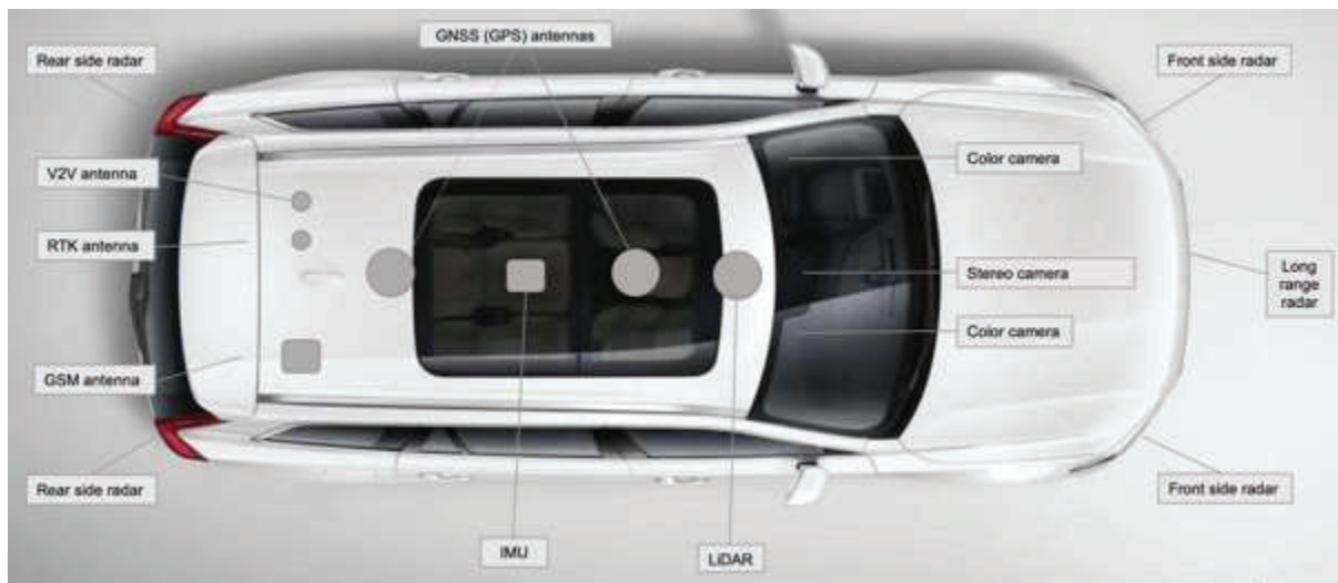
Figur 4. Exempel på ett perceptionssystem på en personbil.
