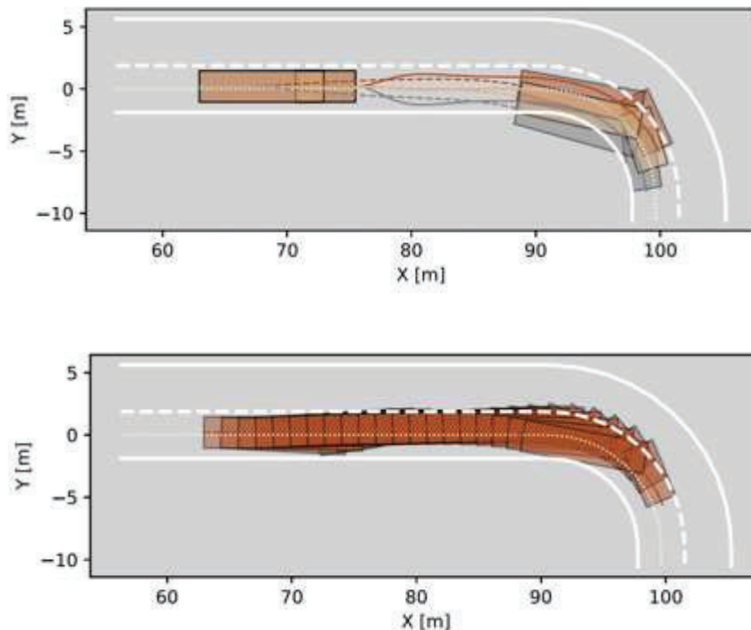
Figur 28. Första och sista iterationen i en serie simuleringar (Nilsson et al, 2018).
