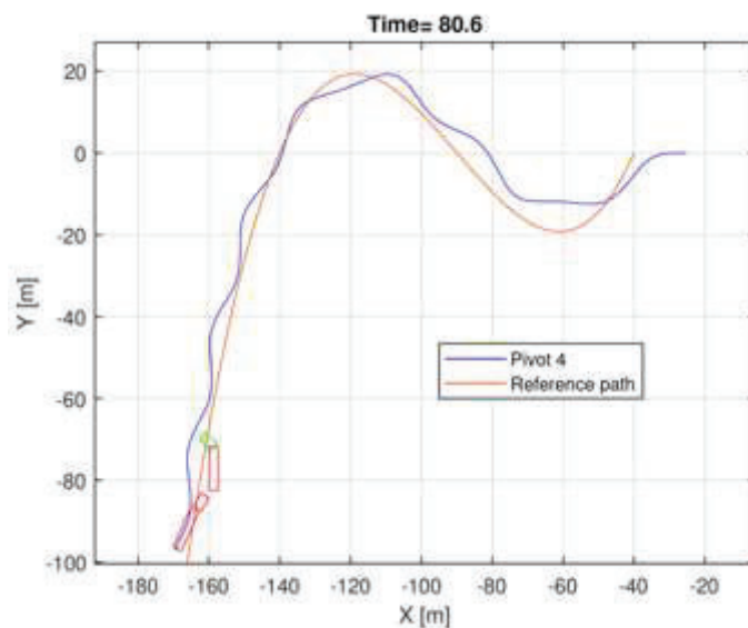
Figur 55. Exempel på simulering av backning längs en viss bågform (Högländer et al, 2021).
