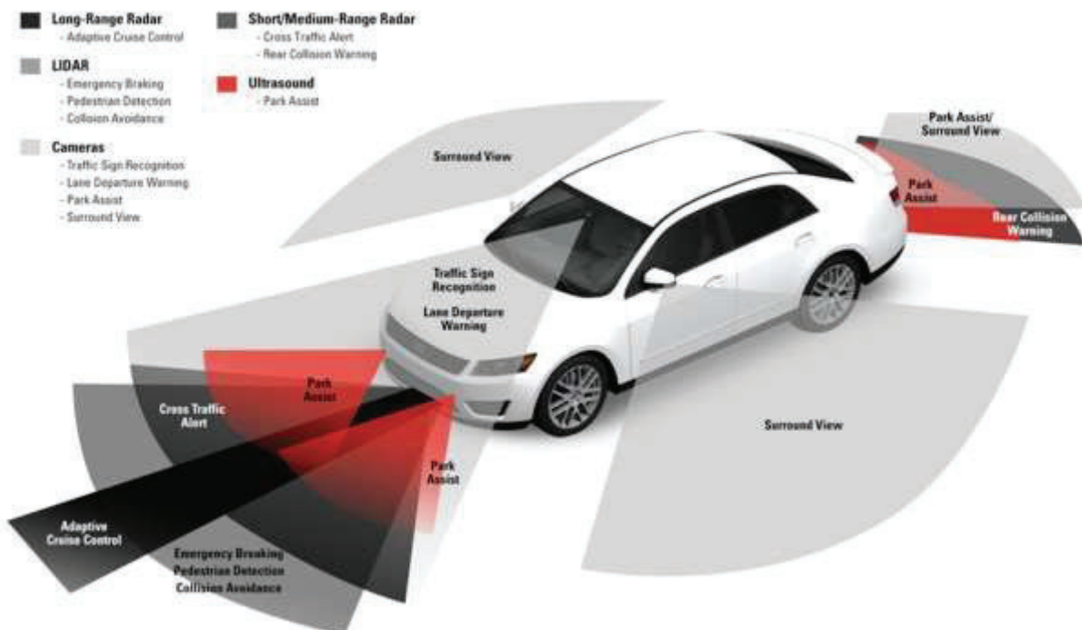
Figur 8. Exempel på avancerade förarstödsystem, ADAS (Francis, 2017).
